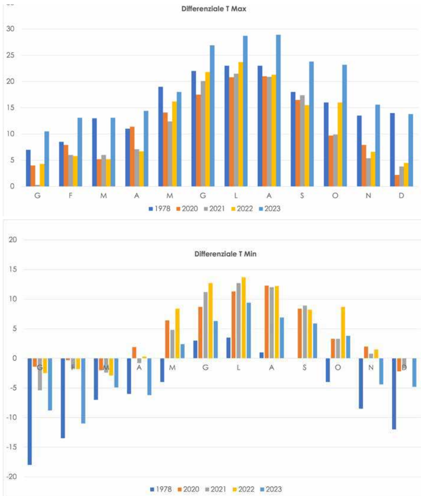
Figura 7 – Grafico andamento temperature MAX per anno (sopra) e temperature MIN per anno (sotto)
