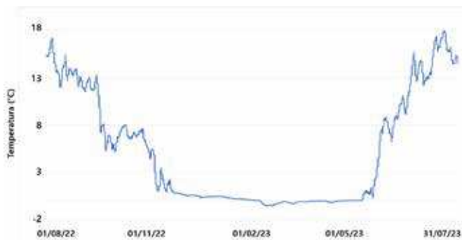
Figura 10 – Grafico dell'andamento della temperatura del suolo relativo al logger L05
