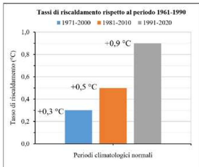
Figura 3 – Tassi di riscaldamento della temperatura dell'aria dei tre precedenti periodi climatologici normali (1971-2000, 1981-2010 e 1991-2020) rispetto al periodo 1961-1990
