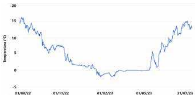
Figura 11 – Grafico dell'andamento della temperatura del suolo relativo al logger L06
