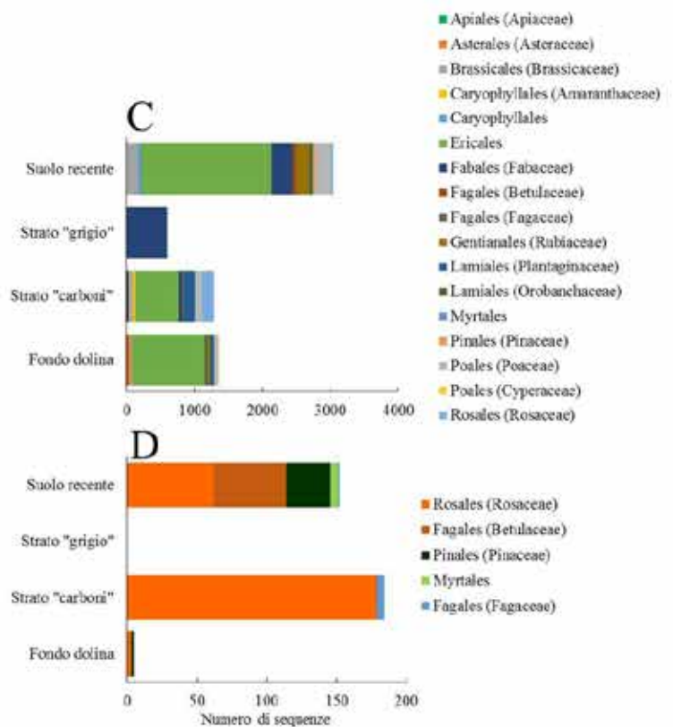
Figura 1 – A - la dolina sommitale del Monte Cervati ubicata a circa 1.850 m s.l.m., oggetto dello studio, durante un'escursione intersezionale campana del CAI (Giugno 2022); B - profilo di campionamento presso la dolina; C - abbondanza di tutti i taxa rilevati mediante sequenziamento del DNA; D - abbondanza dei soli taxa appartenenti a specie arboree. Notare i fori rotondeggianti generati durante il campionamento di suolo - ph Giuliano Bonanomi
