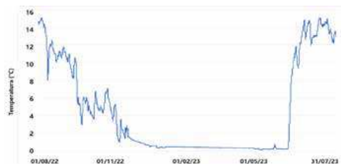
Figura 7 – Grafico dell'andamento della temperatura del suolo relativo al logger L02
