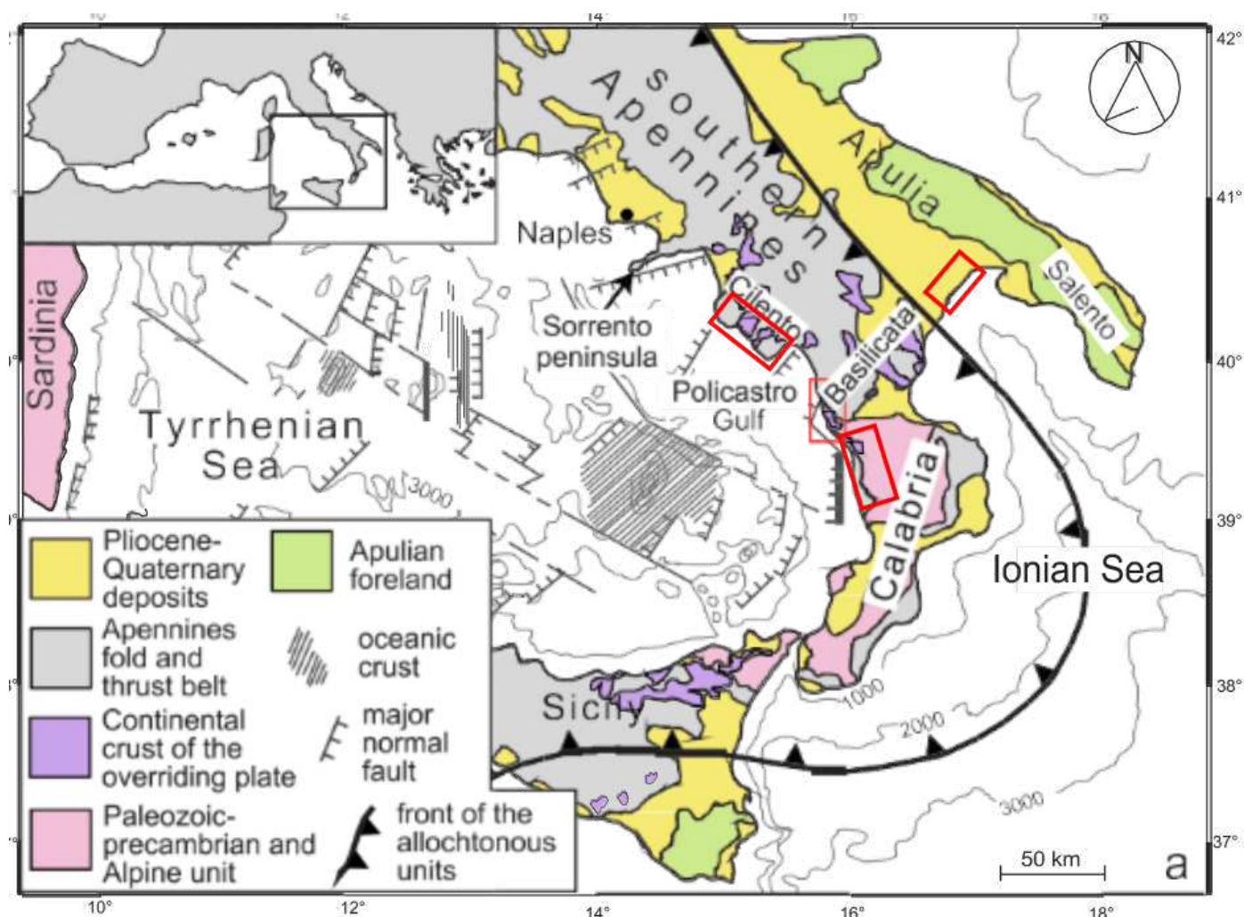
Figura 2 – Schema tettonico semplificato del bacino di retro-arco del Mar Tirreno e della fascia montuosa dell'Appennino meridionale (ridisegnato e modificato da Moussat et al., 1986)
