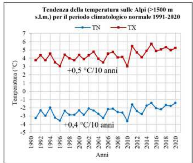
Figura 2 – Tendenza della temperatura minima (TN) e massima (TX) annuale negli ambienti alpini di alta quota (>1500 m s.l.m.) osservata per il periodo climatologico normale 1991-2020
